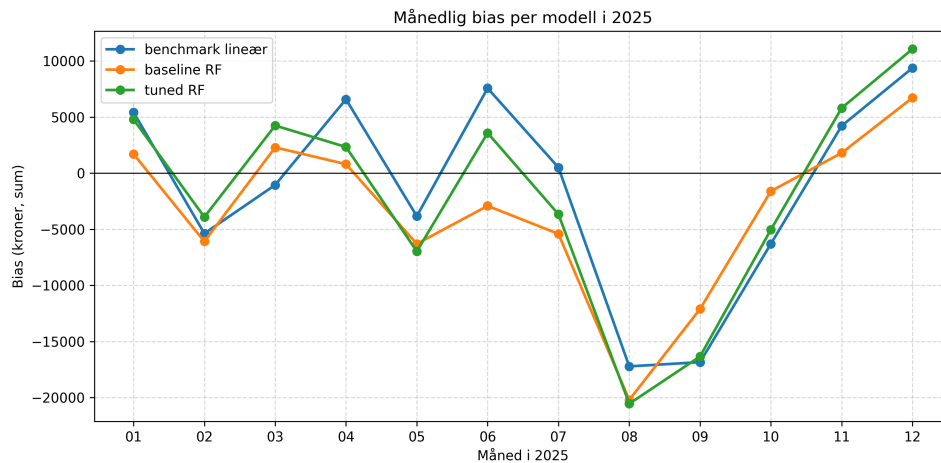
Figur 8: Figur 7.1 Månedlig bias per modell i 2025. Positive verdier betyr at modellen overestimerer salget, negative at den underestimerer. Kurven viser at alle tre modellene underestimerer i august–september.
