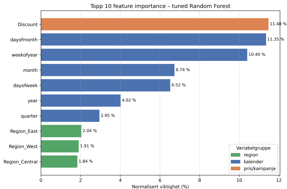
Figur 11: Figur 8.2 Topp 10 feature importance for tuned Random Forest. Variablene er rangert etter normalisert viktighet og viser hvilke signaler modellen faktisk vektlegger.
