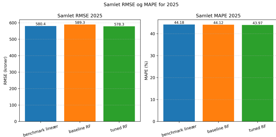
Figur 10: Figur 8.1 Samlet RMSE og MAPE for benchmark lineær, Random Forest baseline og tuned Random Forest i 2025. Tuned Random Forest har lavest RMSE, mens MAPE er tettere fordelt mellom modellene.
