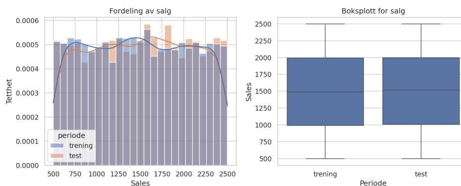
Figur 7: Figur 5.2 Fordeling av daglige salgsverdier i trenings- og testperioden. Overlappet i fordelingene tyder på at målvariabelen er stabil mellom periodene.
