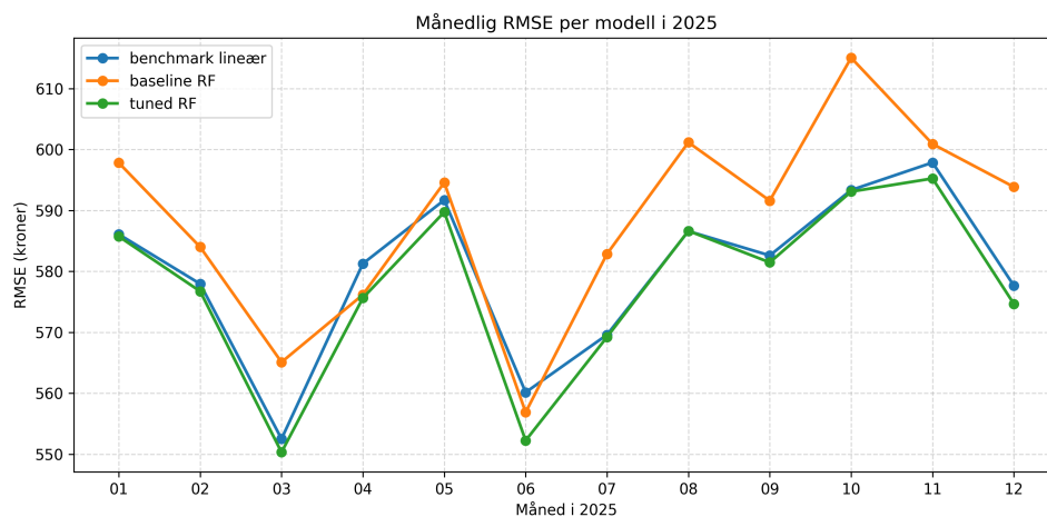
Figur 9: Figur 7.2 Månedlig RMSE per modell i 2025. Tuned Random Forest har lavest RMSE i majoriteten av månedene, mens benchmark lineær slår gjennom i enkeltmåned.
